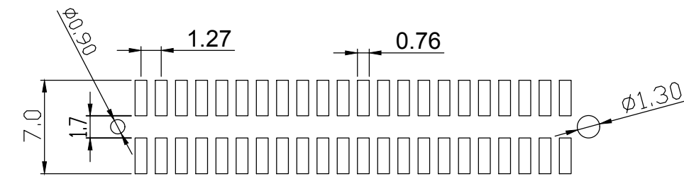
P.C.B Layout
