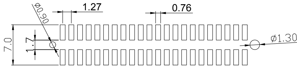
P.C.B Layout
